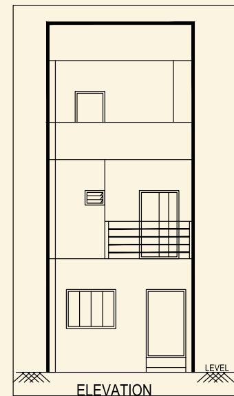
ELEVATION ELEVATION
