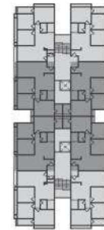
L-M-N-O BLOCK 3 BHK - TYPE 12
